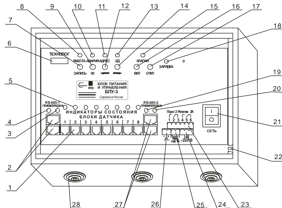
Рисунок 1 – Внешний вид БПУ-3 (БПУ-4)
